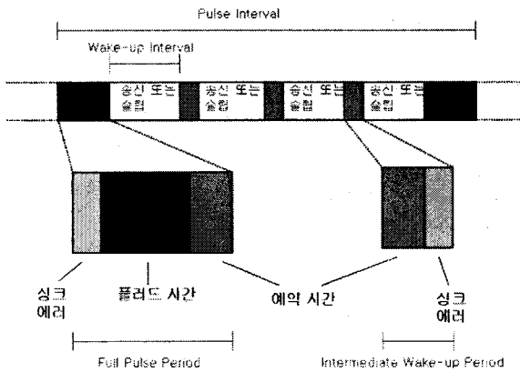
그림 1. PULSE 프로토콜의 동작
