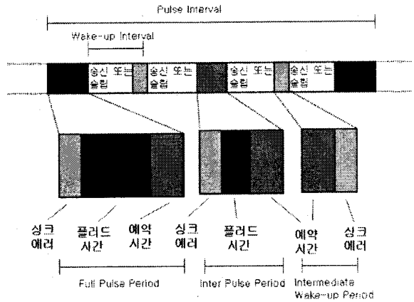
그림 2. M-PULSE 프로토콜의 동작
