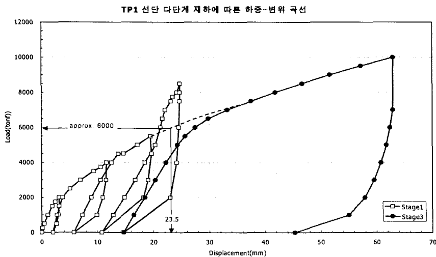
그림 4. 다단계 재하에 의한 선단하중-변위 곡선 해석 일례 (인천대교 국고구간)
