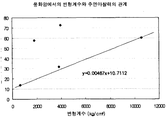
(b) 변형계수와 주면마찰력
