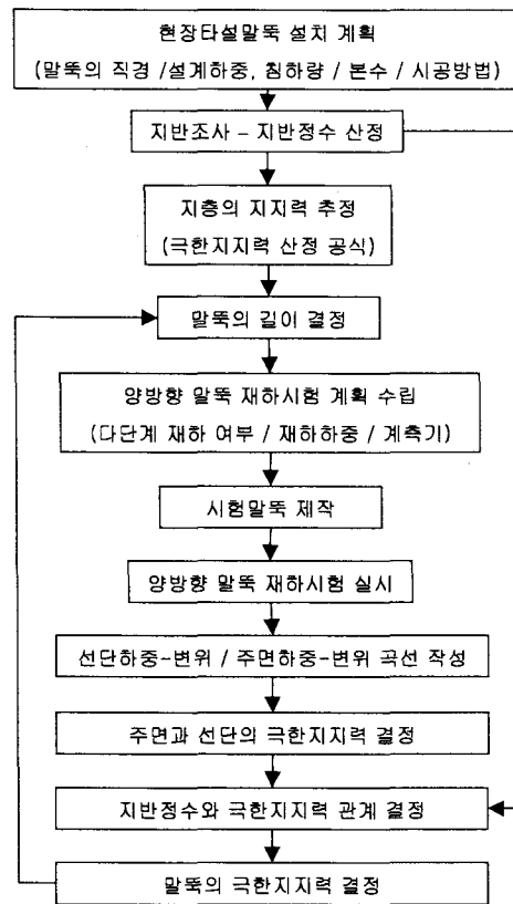
그림 1. 양방향 말뚝 재하시험에 의한 연직지지력 산정 순서도
