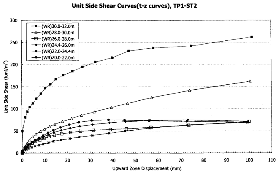
그림 3. 풍화암층에 대한 주면마찰력-변위 곡선(f-w 곡선)의 일례 (인천대교 국고구간)
