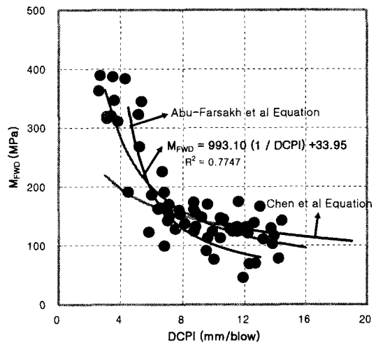
그림 2. DCP-M FWD 의 회귀분석결과와 관계식 비교
