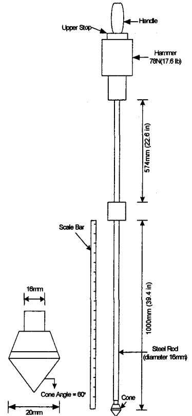
그림 1. 동적 콘 관입 실험(DCP)
