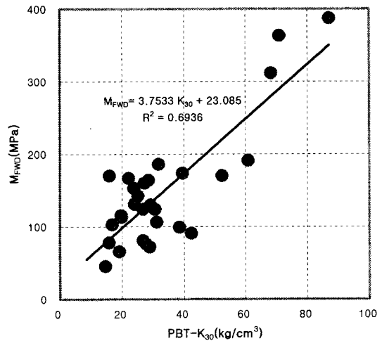
그림 6. K 30 -M FWD 회귀분석결과
