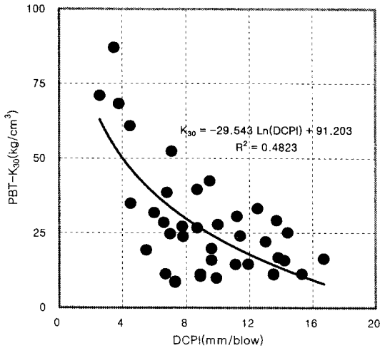
그림 5. DCPI-K 30 회귀분석결과
