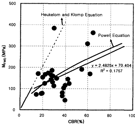
그림 3. CBR-M FWD 회귀분석결과
