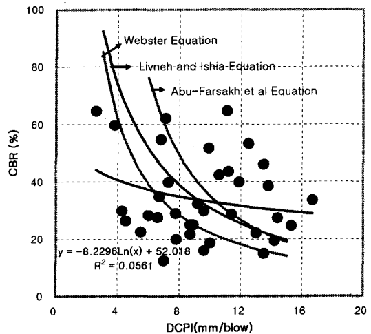
그림 4. CBR-DCPI 회귀분석결과
