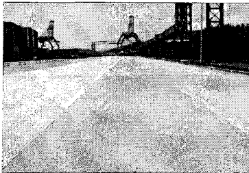
그림 4. 굵은골재 이탈
