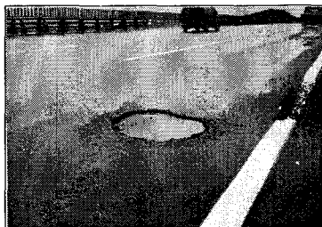
그림 2. 포트홀그림
