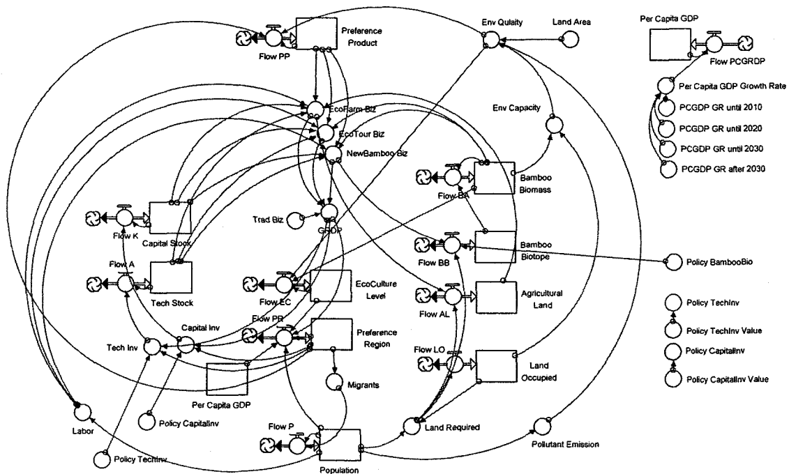
[그림 7] 담양군 실험모형(Stock-Flow Diagram)의 구조
