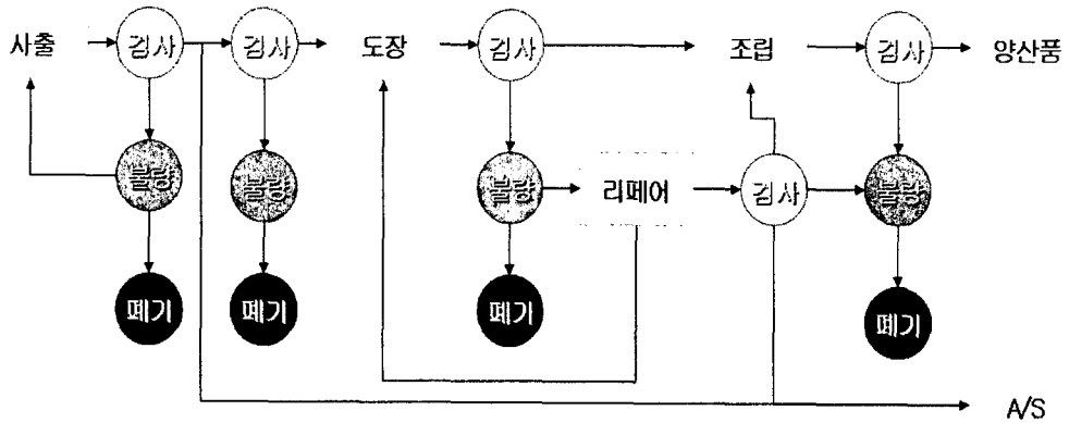
<그림 1> 대상 업체의 주요 공정 흐름도
