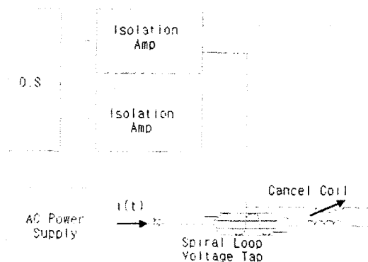
<그림1> 전송전류손실 측정회로
