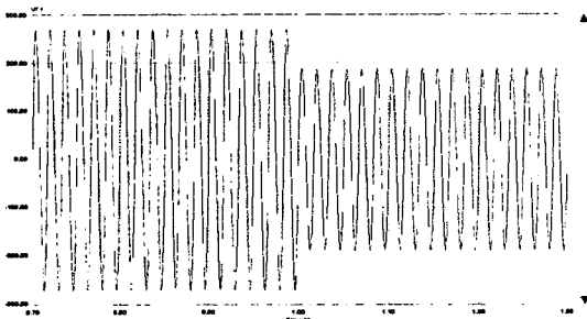
〈그림 6〉 풍력발전기 1대 지락사고시 파형
