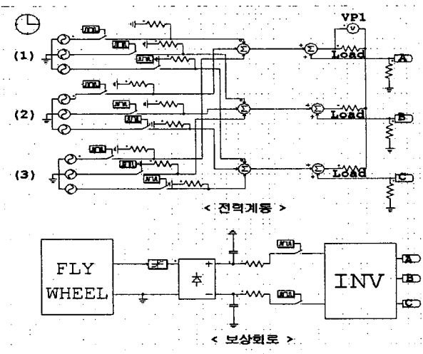
〈그림 5〉 전력안정화시스템 회로도
