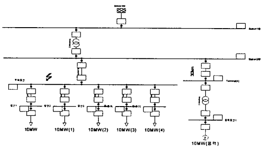
〈그림 2〉 풍력발전단지 연계계통의 단선도
