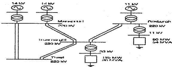
〈그림 3〉 테스트 교류 시스템
