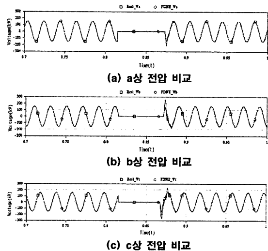
〈그림 6〉 실제 시스템과 FDNE의 전압 비교(고장)
