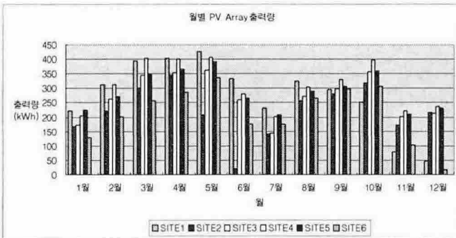
그림 2. 월별 PV 어레이 출력량(kWh)
