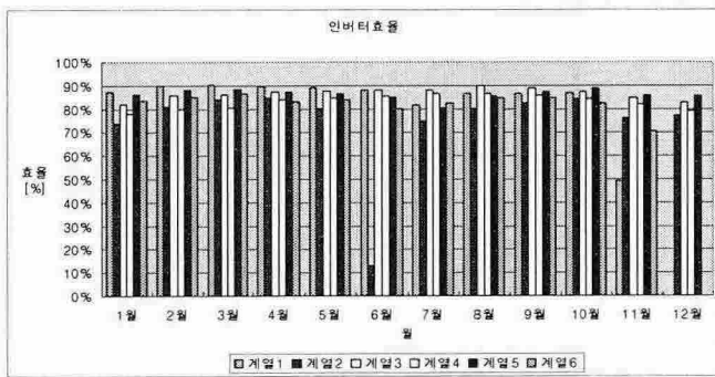
그림 5. 인버터 효율(%)
