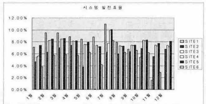
그림 4. 시스템 발전효율(%)
