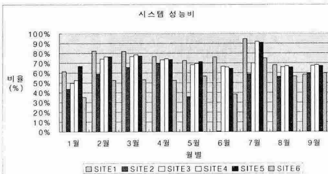
그림 6. 시스템 성능비(%)
