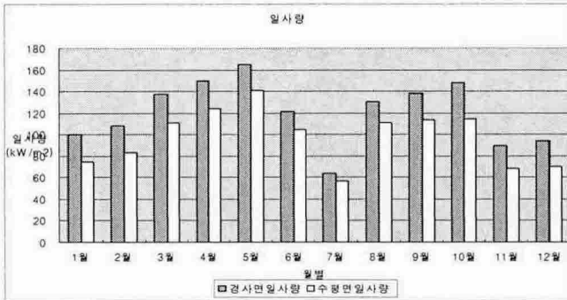
그림 1. 경사면일사량과 수평면일사량
