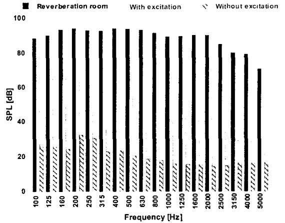
Figure 3 잔향실과 반무향실의 스펙트럼
