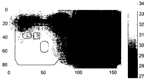
Fig.4 Dash panel 의 투과 손실 분포
