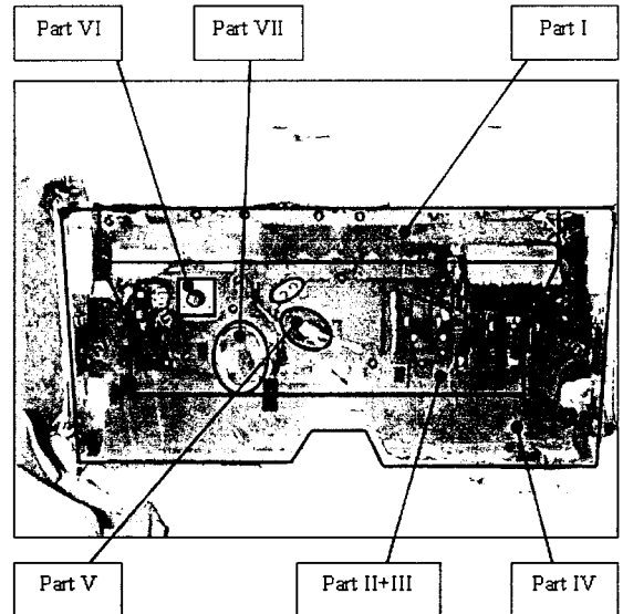
Fig. 6 Dash panel 전면부
