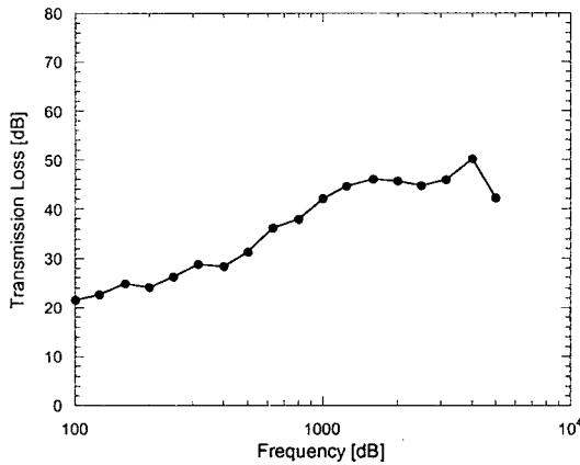
Fig.5 Dash panel 의 투과 손실
