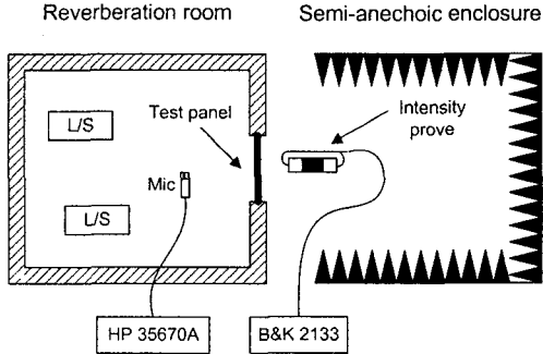
Figure 1 실험장치 구성도
