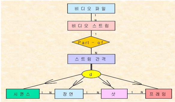
(그림 3) 비디오 소스의 E-R 다이어그램
