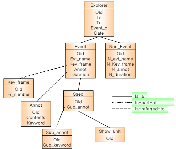
(그림 2) 교양 비디오 영역의 클래스 구조
