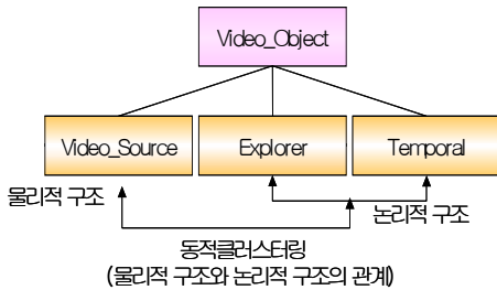
(그림 1) 객체와 클래스 구조
