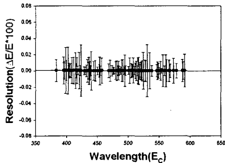
그림 2. Spectrometer의 분해능
