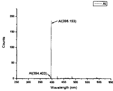
그림 3. Aluminum spectrum
