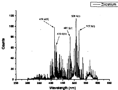
그림 1. Zirconium spectrum
