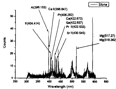
그림 6. 지층굴착 시료 spectrum
