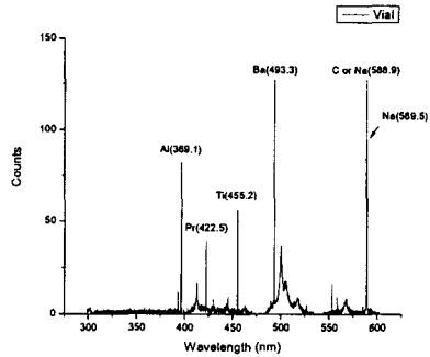
그림 4. Vial spectrum
