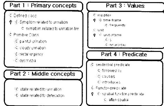
〈그림 4〉 Components of our ontology
