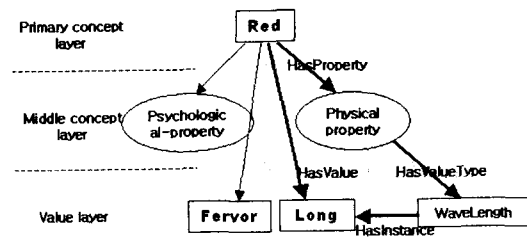
〈그림 8〉 Framework of middle concept
