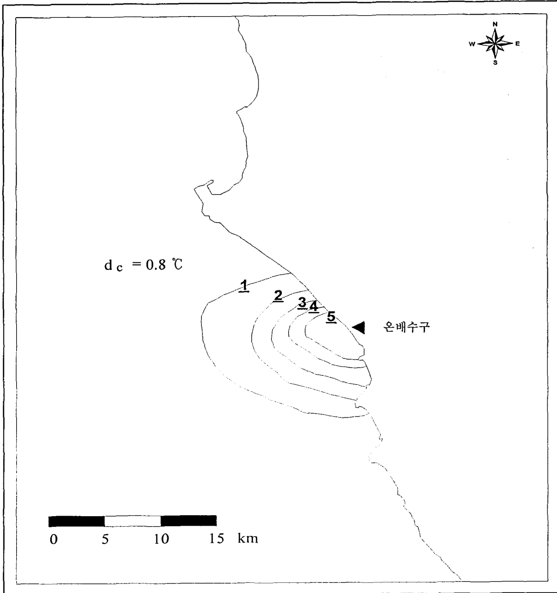
그림 3 발전소 온배수로 인한 온도상승
