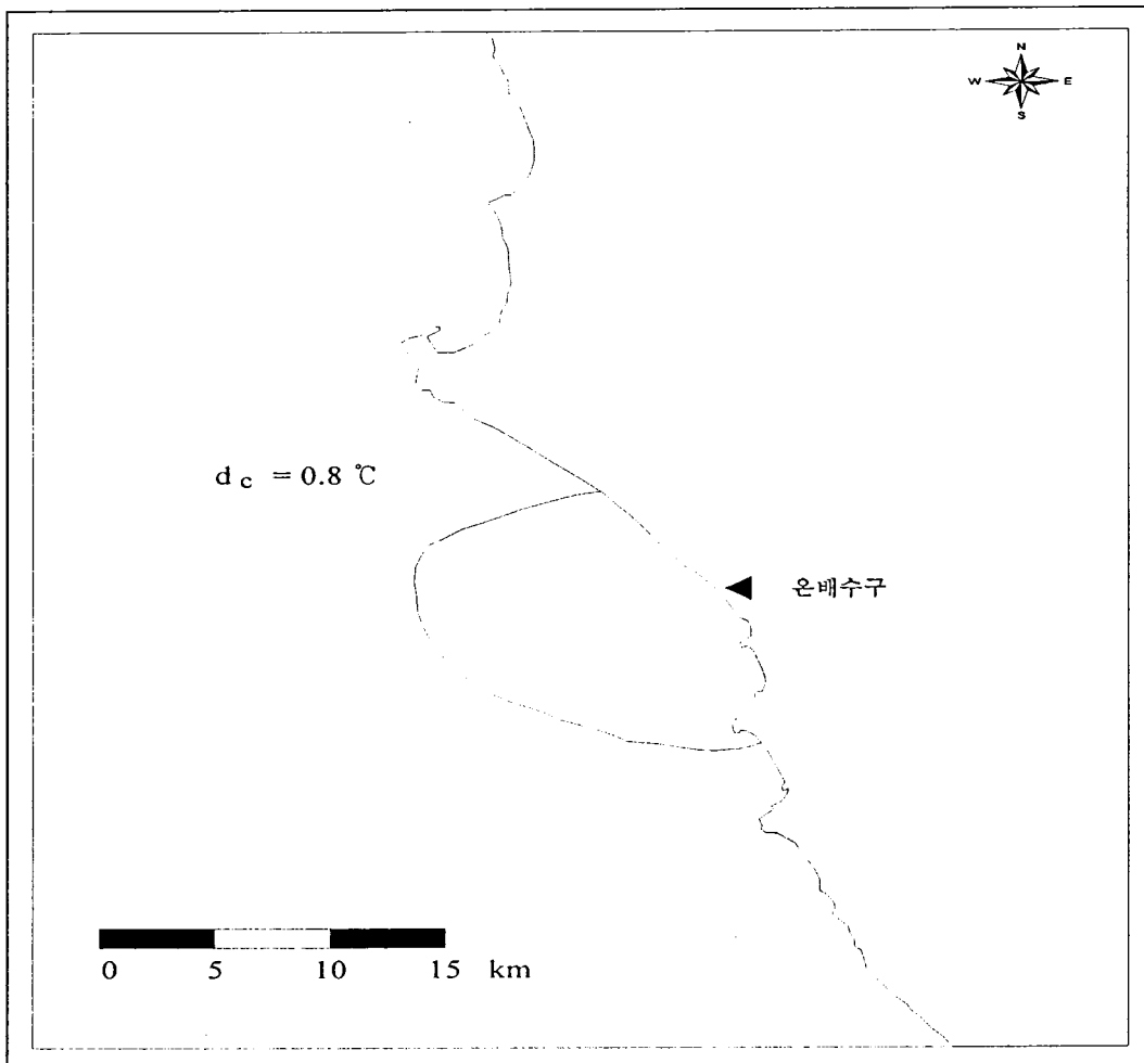
그림 2 발전소 온배수로 인한 어업피해 범위( d_c = 0.8\text{ }^{\circ}\text{C} )
