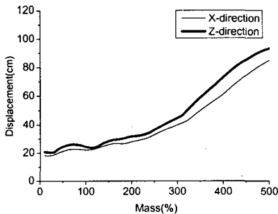
그림 6. 면진층 도입 전 하부구조의 질량 변화에 의한 상부 돔 구조의 변위 응답
