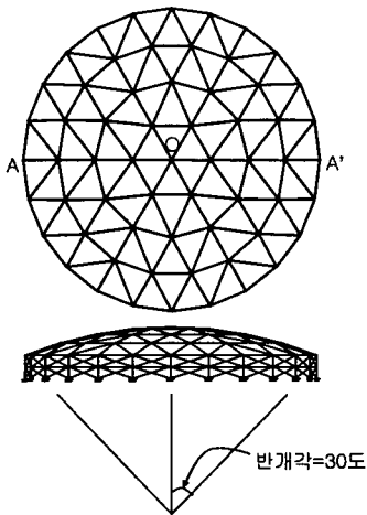
그림 3. 해석 모델
