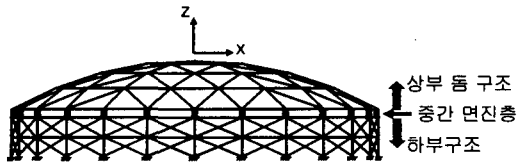
그림 8. 중간 면진층을 도입한 대공간 구조 시스템
