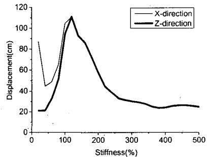
그림 7. 면진층 도입 전 하부구조의 강성 변화에 의한 상부 돔 구조의 변위 응답
