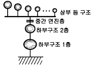
그림 9. 중간 면진층 도입한 등가 모델
