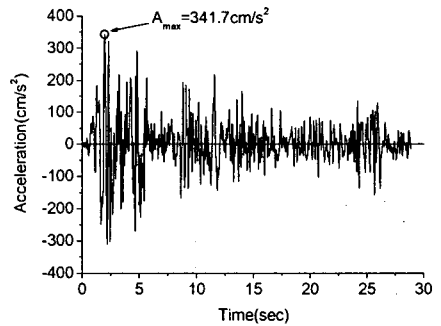
그림 4. 입력지진파(El-Centro NS)
