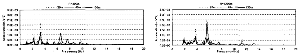
그림 5. 기존열차 곡선부 거리별 가속도주파수 응답
