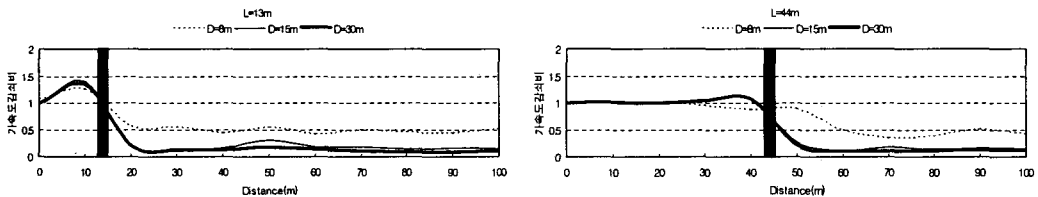
그림 15. 복층에서의 방진구에 의한 가속도 진폭감쇠비(L=13, 44m)
