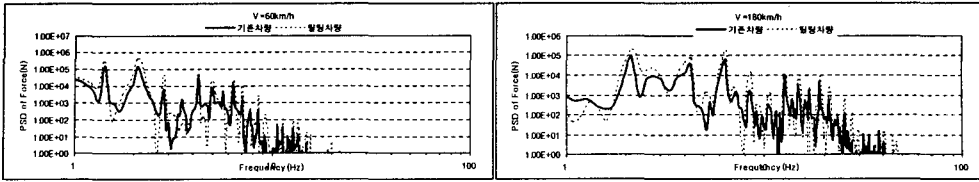
그림 2. 열차주행속도에 따른 전달하중 PSD(침목)
