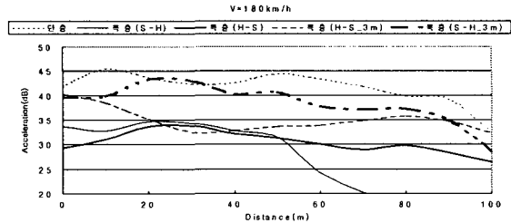
그림 13. 최대 가속도 진폭 감쇠곡선
