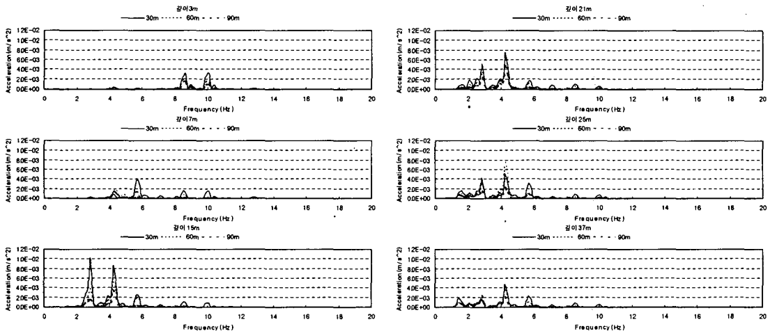
그림 11. 연성지반 깊이에 따른 가속도 주파수 응답
