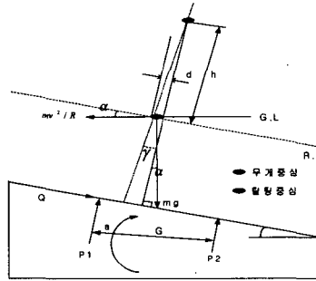
그림 3. 곡선부에서의 틸팅차량의 무게중심에 대한 평형관계
