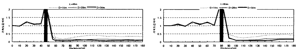
그림 14. 단일층에서의 방진구에 의한 가속도 진폭감쇠비(L=46, 80m)
