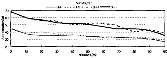
그림 8. 최대 가속도 진폭 감쇠곡선
