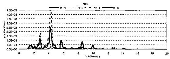
그림 9. 가속도 주파수 응답
