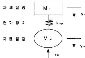
그림 1. 2중질량 차량모형
