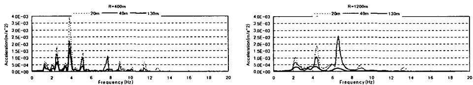
그림 6. 탈팅열차 곡선부 거리별 가속도주파수 응답
