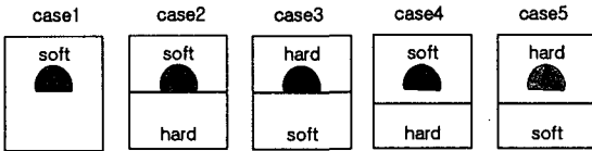
그림 12. 터널위치
