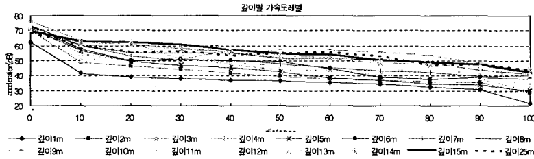
그림 10. 연약층 깊이에 따른 최대 가속도 진폭 감쇠곡선
