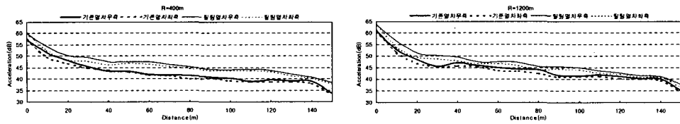
그림 4. 곡선부 거리에 따른 가속도 감쇠곡선
