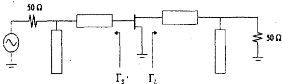
<그림 1> 1단 LNA matching 구조
