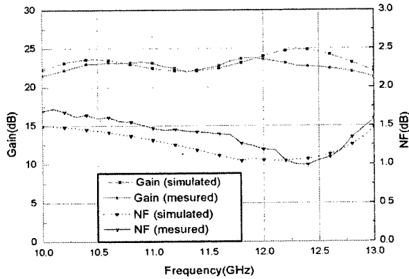
그림 3. Gain 과 Noise Figure의 시뮬레이션 결과와 제작품의 측정치 비교
