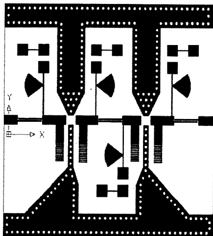
그림 2. LNA의 레이아웃 Fig. 2. 2-stage LNA lay-out
