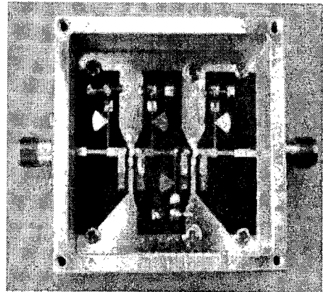
그림 3. 2단 LNA의 제작품 Fig. 3. 2-stage LNA using Microstrip
