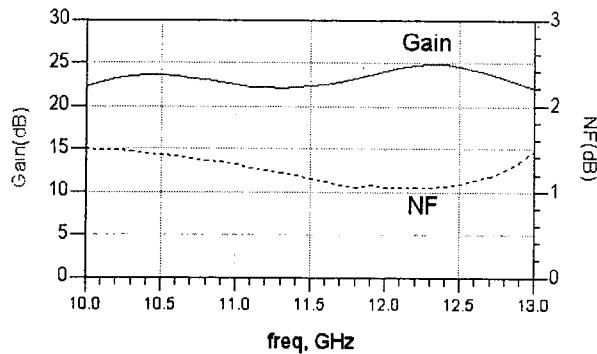
그림 1. Gain과 NF의 시뮬레이션 결과 Fig. 1. Simulation of Gain and NF
