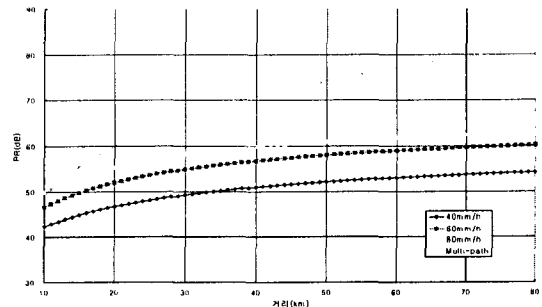
그림 8. 11 GHz에서 보호비 Fig. 8. Protection ratio at 11 GHz.
