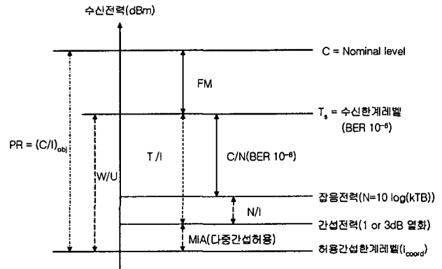
그림 3. 보호비의 도식적 개념
