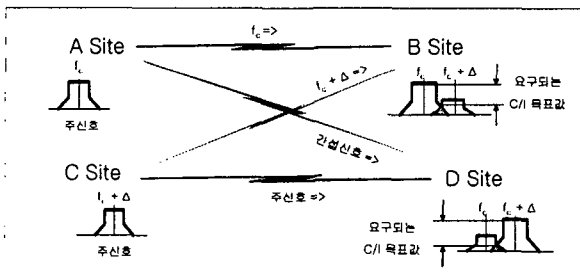
그림 2. 인접채널 간섭
