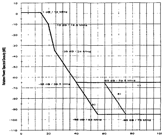
그림 6. 40 MHz 채널의 송신 스펙트럼 마스크 Fig. 6. Tx spectrum mask with 40 MHz channel.
