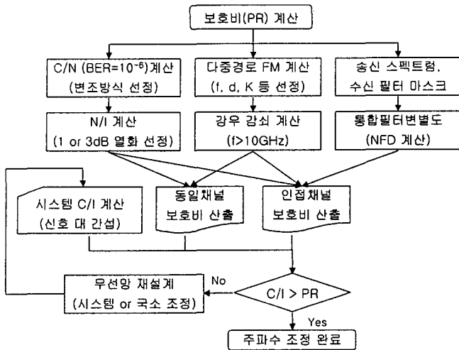
그림 4. 보호비 산출 알고리즘
