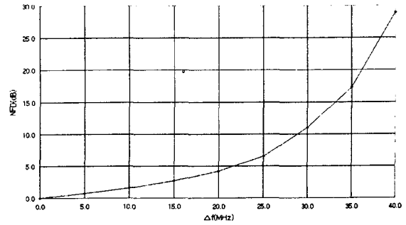
그림 7. 채널 대역폭 40 MHz의 NFD Fig. 7. NFD with channel bandwidth of 40 MHz.
