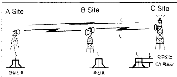
그림 1. 동일채널 간섭
