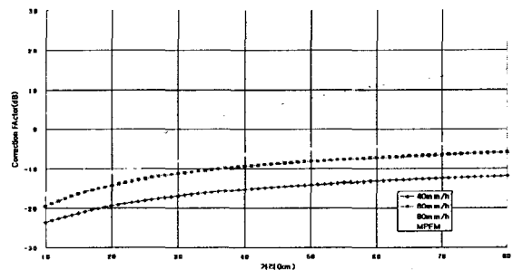
그림 9. 주파수 11GHz에서 보호비 정정인자 Fig. 9. Protection ratio correction factor at 11GHz.
