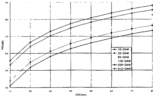
그림 5. 6.7 GHz에서 보호비 Fig. 5. Protection ratio at 6.7 GHz.
