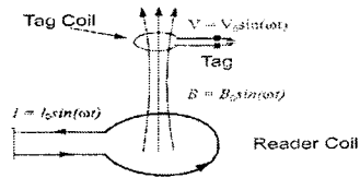
그림 4. 무선 안테나 전압유도 원리
