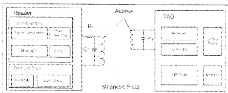
그림 1. 통신모듈 구성도
