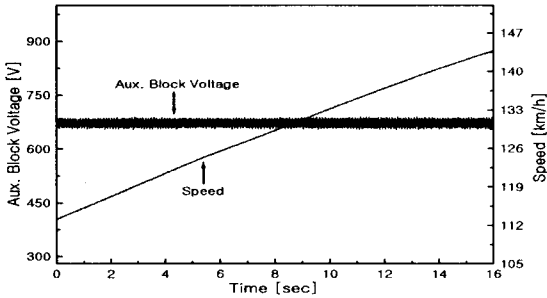
그림 5. 정상시의 보조전원장치 출력전압
