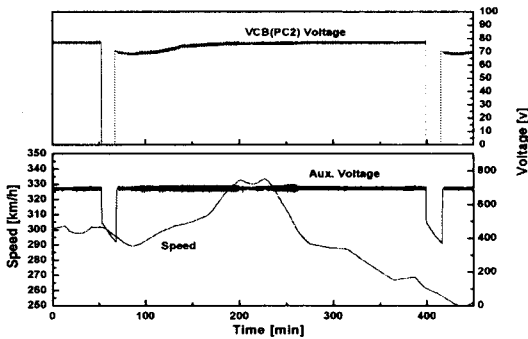
그림 6. 330km/h에서의 Aux. Block 출력전압
