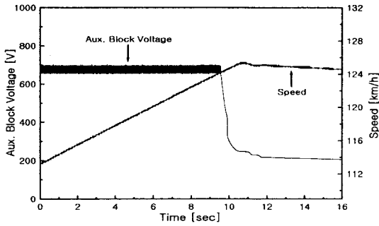
그림 4. 보조전원장치 고장시의 속도 파형
