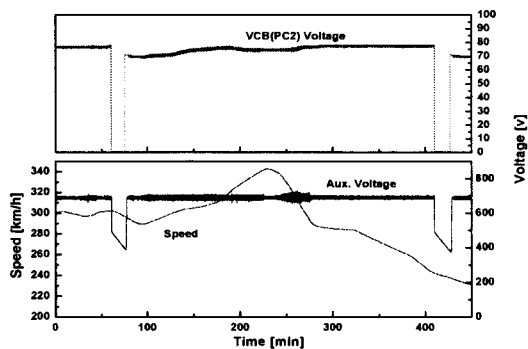
그림 7. 340km/h에서의 Aux. Block 출력전압
