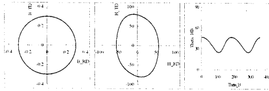
(a) 등방성 시료A, B=0.3T
