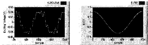
(c) After B Waveform control(이방성 시료C, RD방향)
