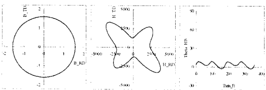
(c) 등방성 시료B, B=1.6T
