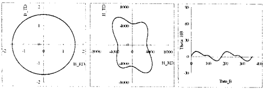
(c) 등방성 시료A, B=1.6T
