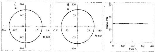
(a) 등방성 시료B, B=0.3T
