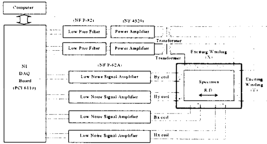
그림 2. 2방향 여자철 Single sheet tester 시스템
