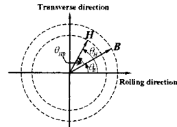
그림 1. 자계의 세기(H)와 자속밀도(B)의 관계
