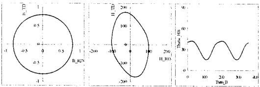
(b) 등방성 시료A, B=0.8T
