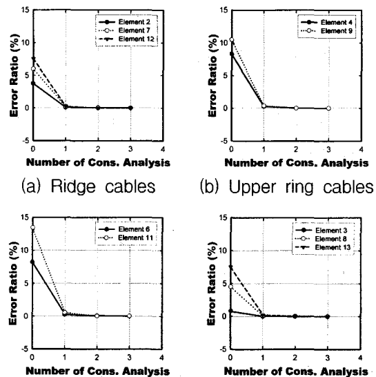
(a) Ridge cables (b) Upper ring cables (c) Lower ring cables (d) Diagonal cables
