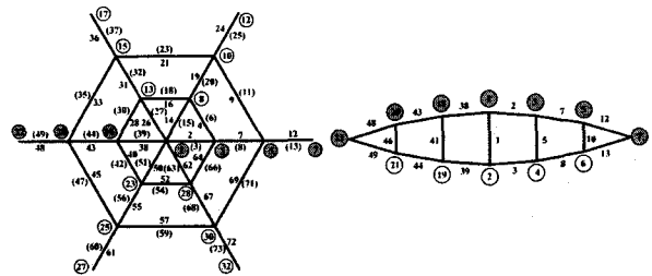
(a) 평면도 (b) 단면도 <그림 3> Zetlin형 케이블 돔
