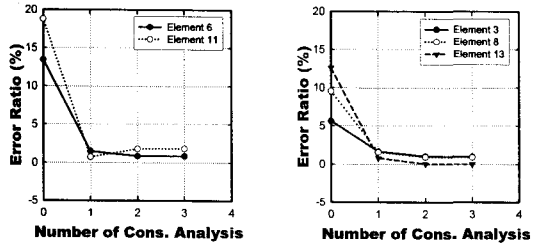
(c) Lower ring cables (d) Diagonal cables
