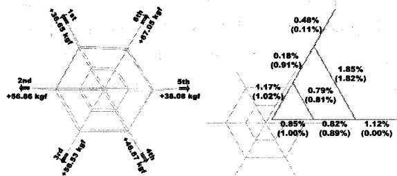
(a) 누적장력량 (b) 부재장력 오차율 <그림 9> 최종시공해석 (Case-2)
