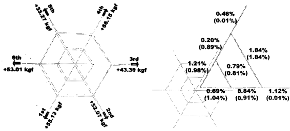
(a) 누적장력량 (b) 부재장력 오차율
