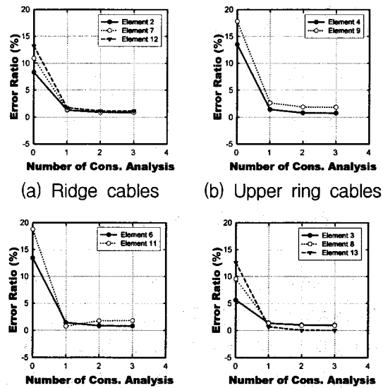
(a) Ridge cables (b) Upper ring cables (c) Lower ring cables (d) Diagonal cables <그림 8> 시공해석 단계에 따른 부재 장력 오차율 (case-2)
