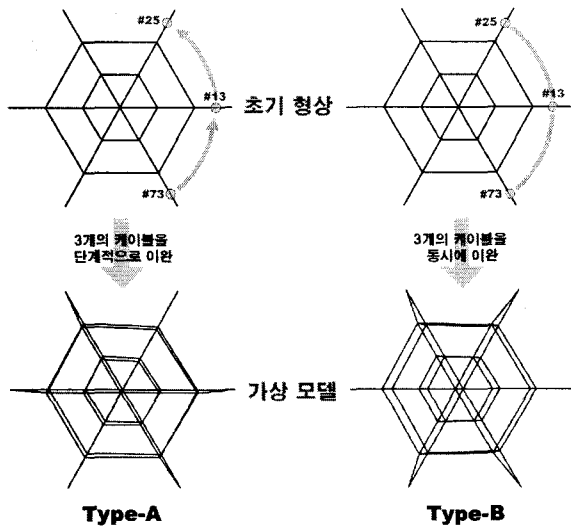
<그림 4> 가상모델의 설정
