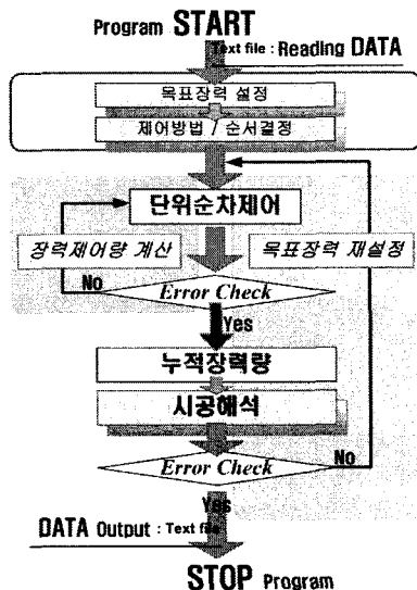
<그림 2> 시공해석의 흐름도
