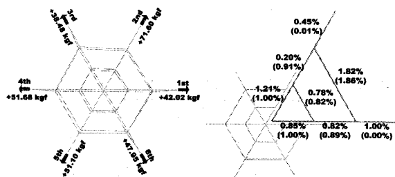
(a) 누적장력량 (b) 부재장력 오차율 <그림 7> 최종시공해석 (Case-1)
