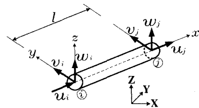
<그림 1> 케이블 요소의 요소 좌표계
