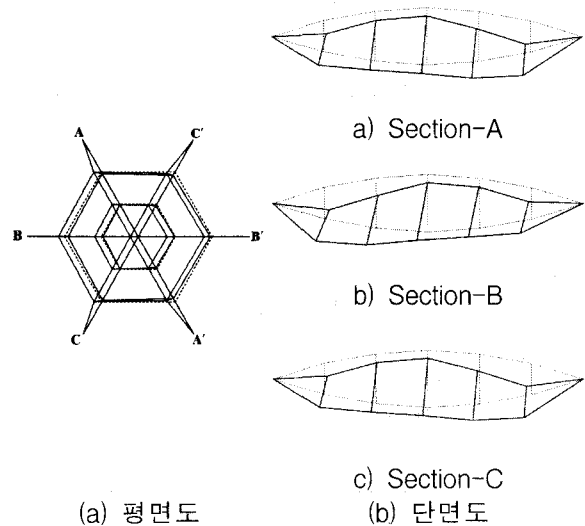
<그림 12> 가상모델 (Type-B, ×300배)
