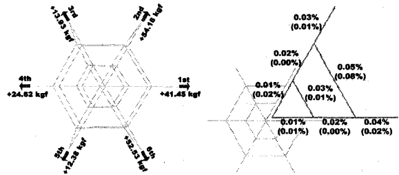
(a) 누적장력량 (b) 부재장력 오차율
