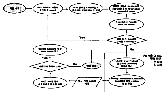
그림 4 MMA간의 협상 알고리즘 흐름도
