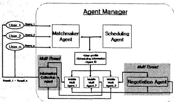
그림 3. Agent Manager 구조도
