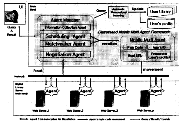
그림 1 본 논문에서 제안하는 MMA 시스템 구조
