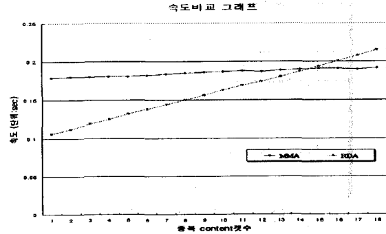
그림 8 속도비교평가 그래프
