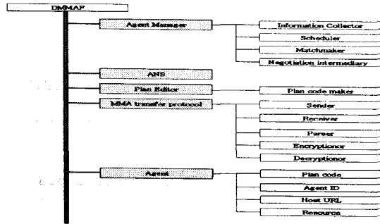
그림 2 DMMAF 구조도
