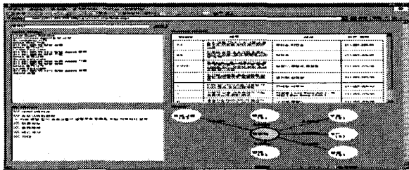
그림 6 최종 검색결과화면
