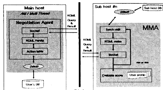
그림 5 MMA와 협상 에이전트간 협상 메카니즘
