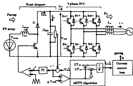
그림 1. 기존의 제안시스템 Fig. 1. existing proposed system
