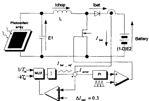
그림 3. 전류제어 Loop Error MPPT controller 회로도 Fig. 3. The circuit of current loop error MPPT controller
