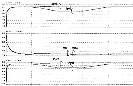
그림 8. 시뮬레이션 파형 Fig. 8. Simulation waveforms
