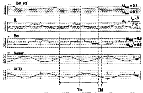
그림 5. 각부의 파형 Fig. 5. Waveform of each part
