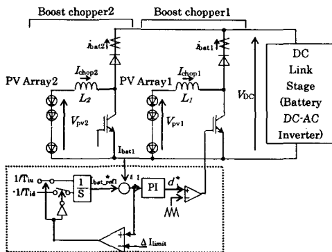
그림 7. 병렬로 다수 연결한 시스템 회로도 Fig. 7. Circuit of parallel connected system
