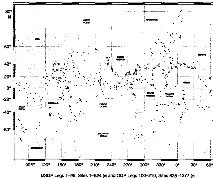
그림 1. DSDP, ODP 시추 위치
