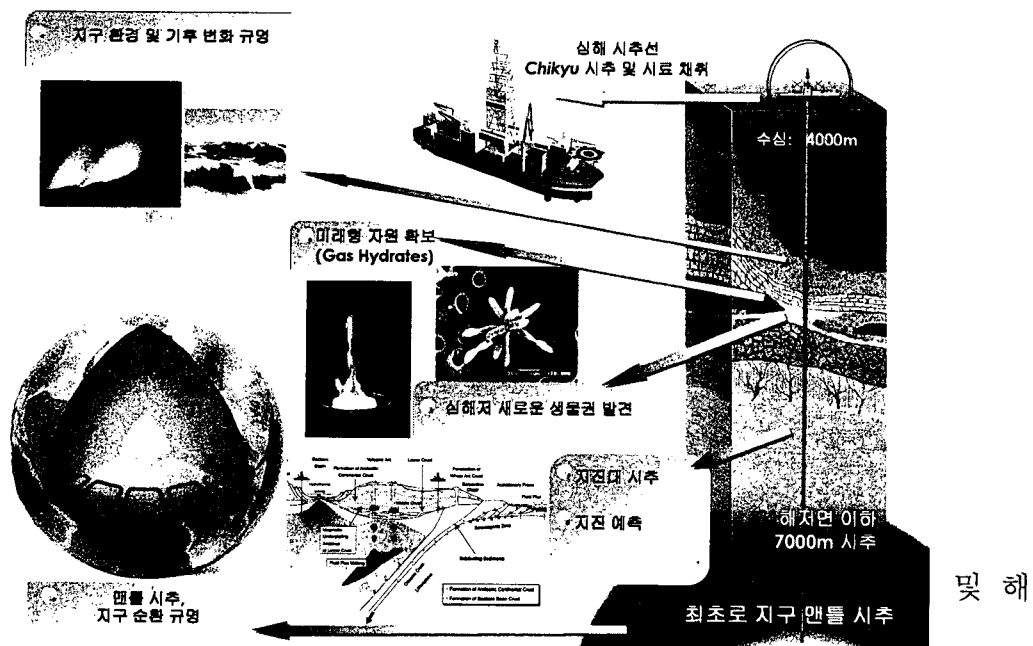
그림 2. 국제공동해양시추사업(IODP)의 주요 연구 분야 및 목적
