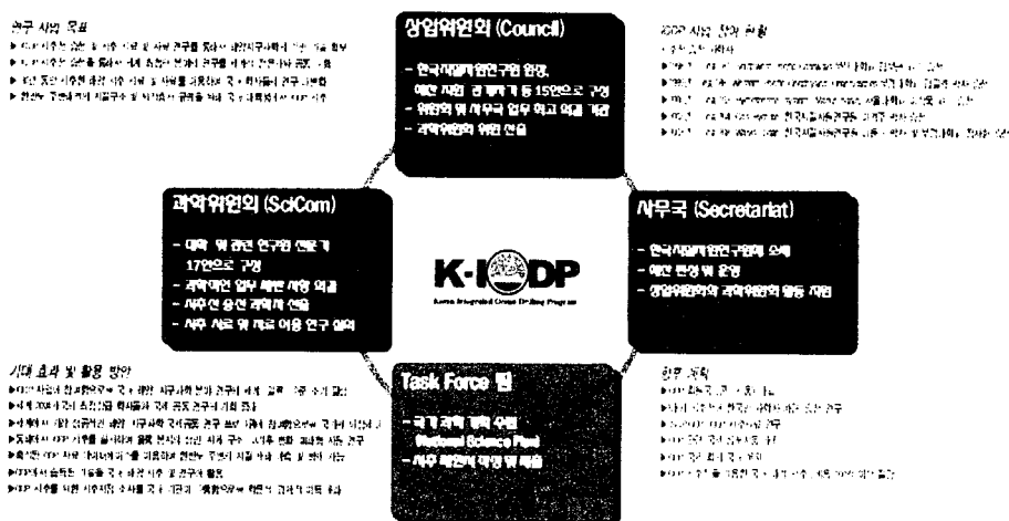
그림 3. 국제공동해양시추 사업의 위원회 및 기구 조직도
