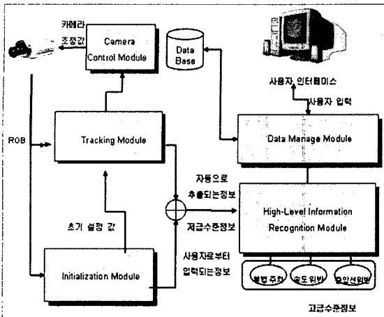
<그림 2-1> 교통 감시 시스템의 전체적인 구조
