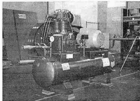
그림 1. 공기압축기의 외형
