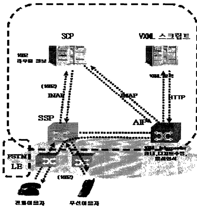
(그림 1) Everlink 1582 음성다이얼 서비스 개요도
