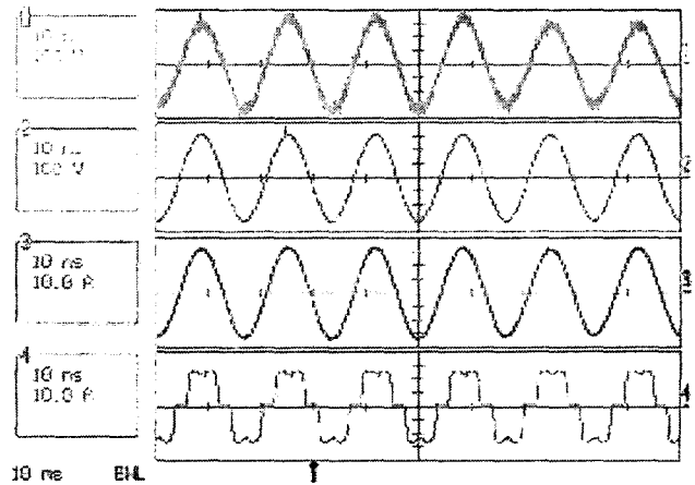
그림 14 전원전압 15% Swell시(63% 비선형부하)
