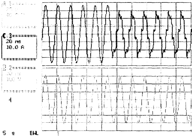
그림 12 비선형부하시 응답(63%부하) 확대
