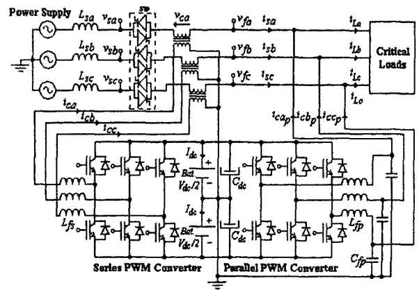
그림 2 델타 변환 UPS 시스템 구성도 Fig. 2 Delta conversion UPS system diagram
