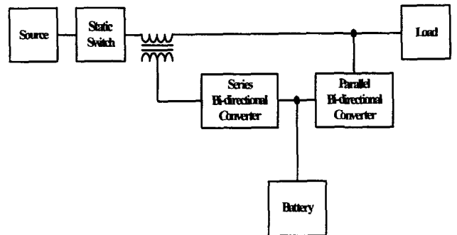
그림 1 델타 변환 방식 Line interactive UPS의 구조 Fig. 1 Structure of delta conversion line-interactive UPS
