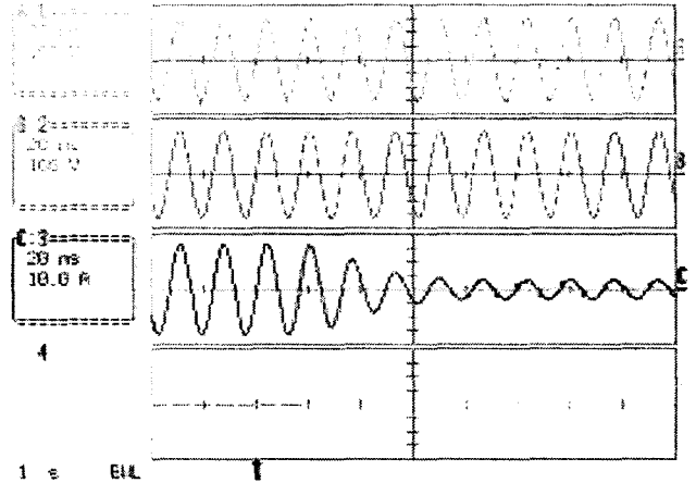
그림 8 비선형부하시 응답(63%→무부하) Fig. 8 Response of nonlinear load(63%→No-load)
