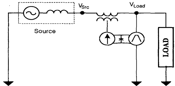
그림 3 델타 변환 UPS 시스템 단상 등가회로도 Fig. 3 Single-phase equivalent circuit diagram of delta conversion UPS system
