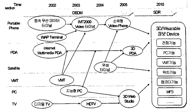
그림 7 통합단말 발전전망
