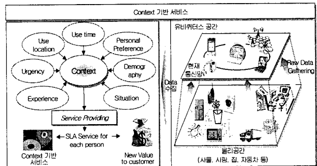
그림 8. Context기반 서비스
