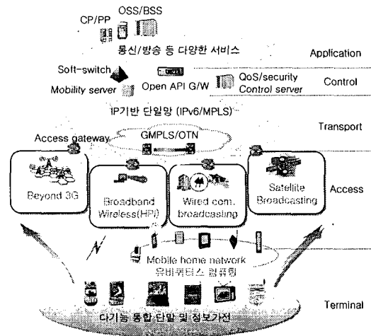
그림 2. BcN 구조
