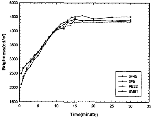
그림 1. 권선수 13회의 시간에 따른 휘도 변화
