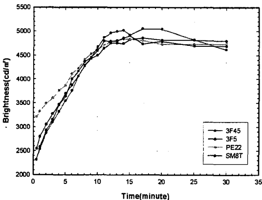
그림 2. 권선수 14회의 시간에 따른 휘도 변화
