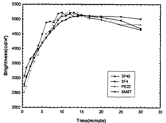
그림 3. 권선수 15회의 시간에 따른 휘도 변화
