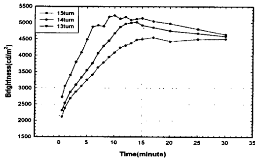
그림 8. 시간과 권선수에 따른 휘도 특성.
