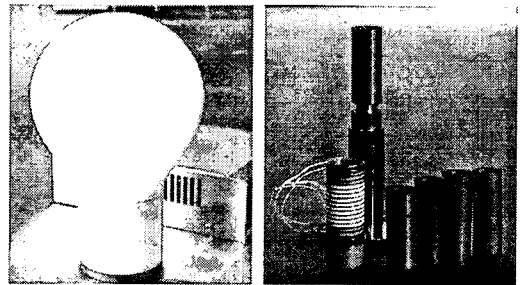
그림 2. 무전극 램프와 안테나.
