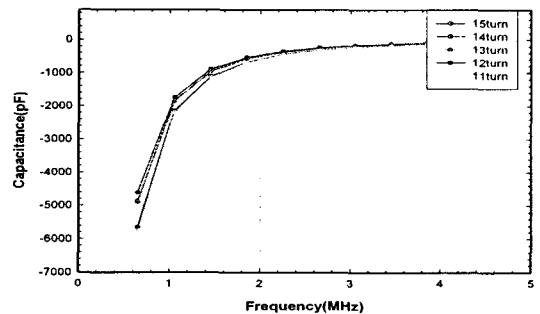
그림 6. 주파수와 권선수에 따른 capacitance 특성.
