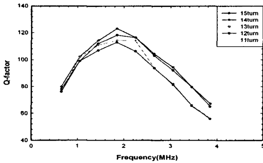
그림 3. 주파수와 권선수에 따른 Q-factor 특성.
