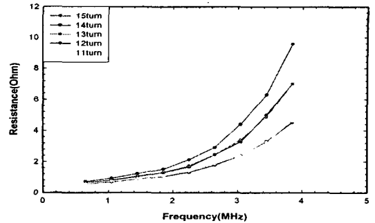
그림 5. 주파수와 권선수에 따른 resistance 특성.
