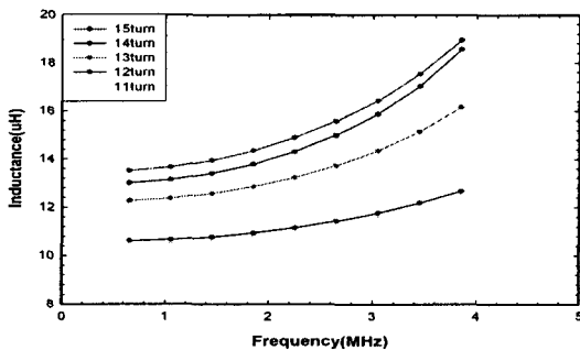
그림 4. 주파수와 권선수에 따른 inductance 특성.
