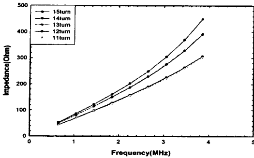
그림 7. 주파수와 권선수에 따른 impedance 특성.
