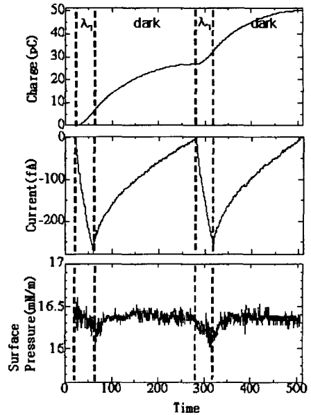
그림 6. AZ-G4의 광조사( \lambda_1=365\text{nm} ) Fig. 6. Photoirradiation of AZ-G4( \lambda_1=365\text{nm} )
