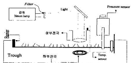
그림 3. 수면위의 광자격 전달에 따른 변위전류 측정장치 Fig. 3. Displacement current measuring apparatus according to light stimulus transfer on water surface
