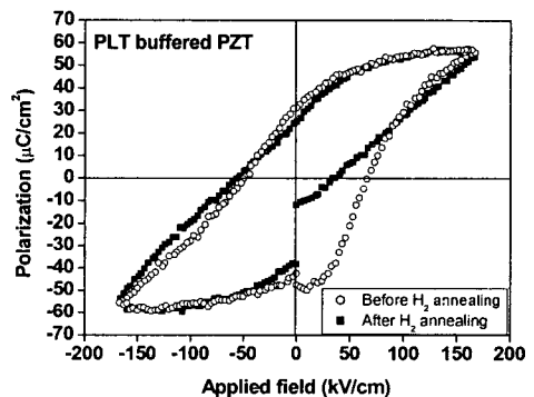
Figure 2. 수소 후열처리 전과 후의 PLT buffer가 증착된 PZT 박막의 hysteresis 특성.
