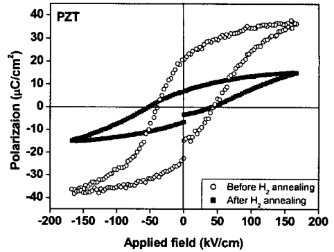
Figure 1. 수소 후열처리 전과 후의 PZT 박막의 hysteresis 특성.
