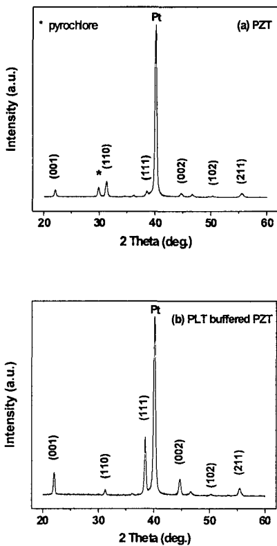
Figure 3. (a) PZT (b) PLT buffer가 사용된 PZT 박막의 XRD pattern.
