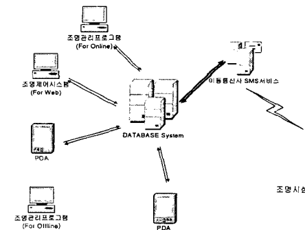
그림 1. 시스템 구성도. Fig. 1. System architecture.
