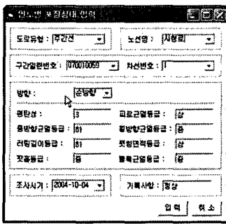
그림 5. 입력창의 예
