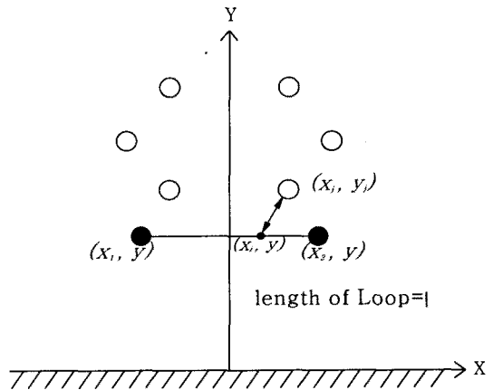
그림 1. 수동 루프를 채용한 송전선로 단면도
