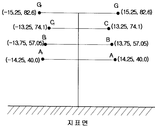
그림 2. 송전선로 상배치 및 지표로부터의 거리
