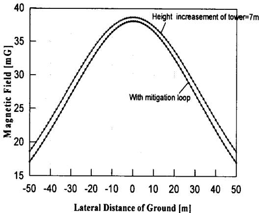
그림 6. 자계 저감 대책 기술에 따른 효과 분석
