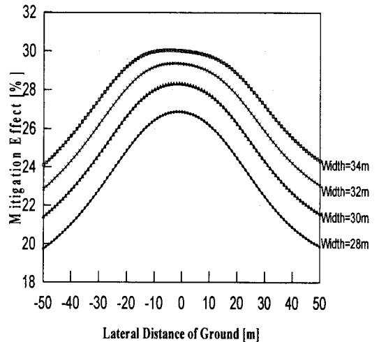
그림 4. 지표면 위 1[m]지점에서의 자계 저감 효과 (루프의 높이 고정=30m)
