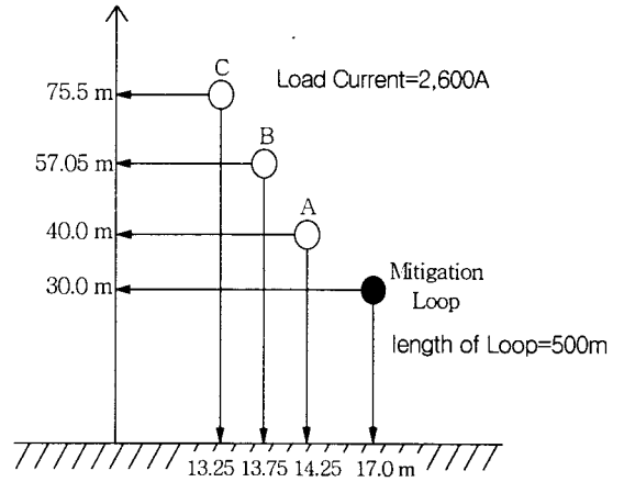
그림 3. 765 kV 송전선로의 기하학적 구조
