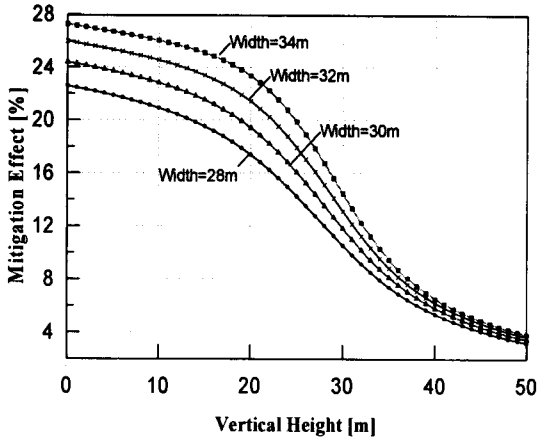
그림 5. 높이에 따른 자계 저감 효과 (루프의 높이 고정=30m, X=30m)
