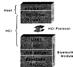
그림 1. Bluetooth protocol stack
