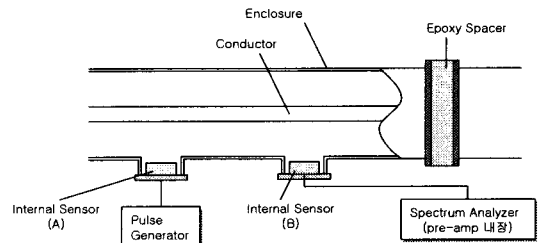
그림 6. Pulse Generator 시험 구성도
