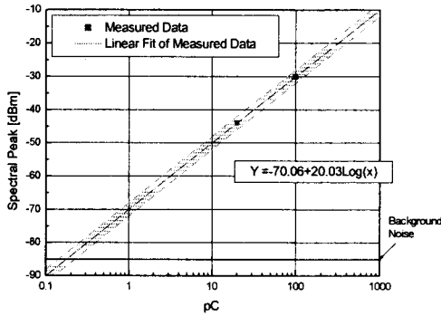
그림 4. UHF 센서 특성 곡선 (시험 데이터)
