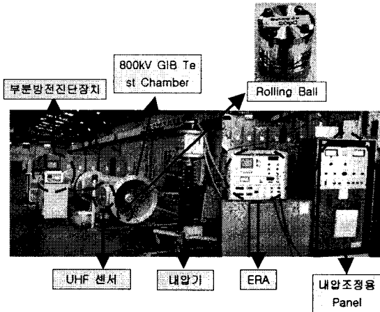
그림 3. UHF 센서특성시험 장비
