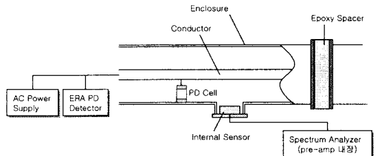
그림 2. UHF 센서 특성시험 구성도
