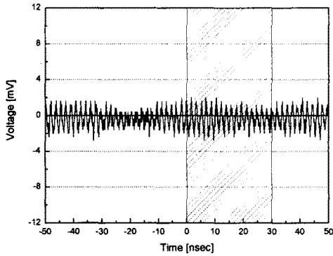
그림 11. 구간 1에서 500V 인가시 측정 결과
