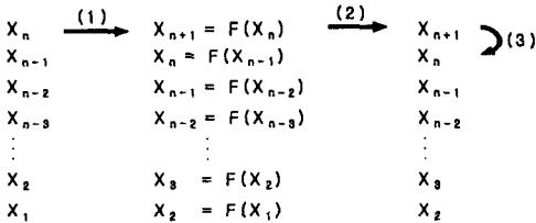
그림 2 기존 일회용 패스워드 매커니즘에서의 일방향 함수 운용 개념
