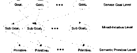
그림1. 상호-주도를 위한 계층적 베이지안 네트워크
