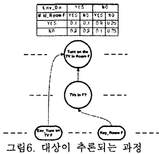
그림6. 대상이 추론되는 과정
