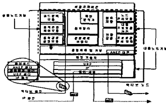
그림 5. 액티브 노드 모델링
