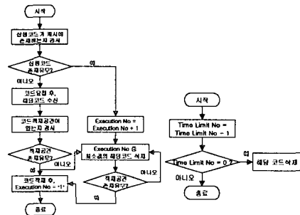
그림 4. 코드 캐싱 기법의 동작 과정
