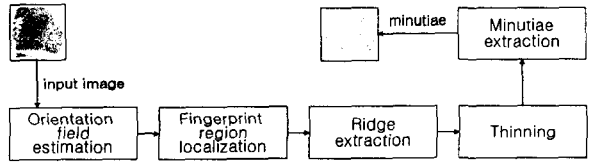
그림 1. 특징점 추출 단계
