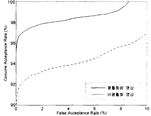
그림 6. 그리드 기반 매칭 알고리즘을 이용한 인식성능 ROC
