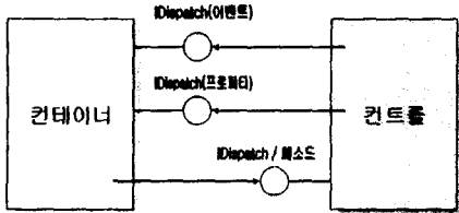
그림 1. ActiveX 컨트롤의 동작 방식
