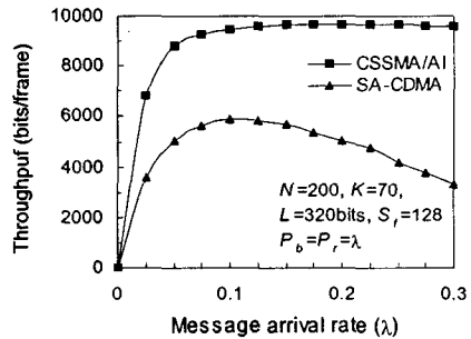
그림 3. 처리율 비교
