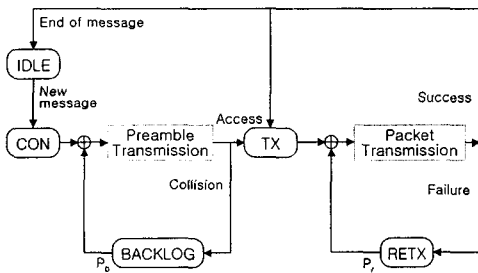
그림 2. 프로토콜 동작
