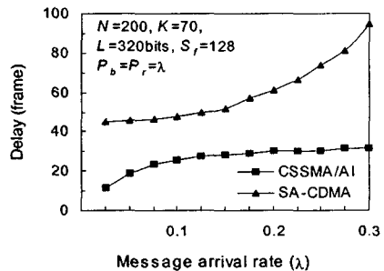
그림 4. 지연 비교
