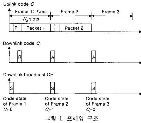
그림 1. 프레임 구조
