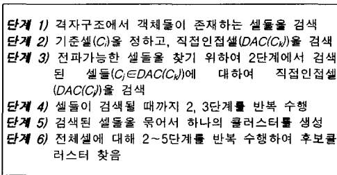
그림 5. 클러스터 생성 알고리즘
