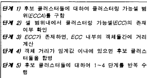
그림 6. 클러스터 합병 알고리즘
