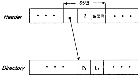
그림 4. 균등격자 구조의 예
