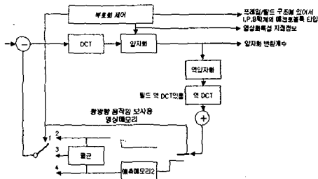
그림 1. MPEG-2의 부호기
