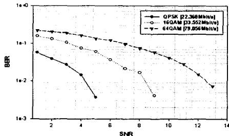
그림 6. AWGN환경에서 변조방식에 따른 BER성능
