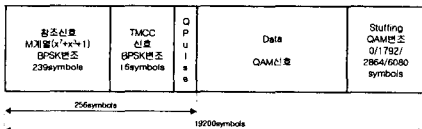
그림 4. 파형등화용 기준신호의 Format
