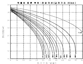
그림 4. 급전선로 P-V 곡선(급전거리 30km)
