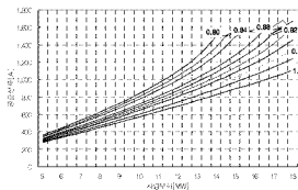
그림 11. 부하, 역률에 따른 변전소 공급전류
