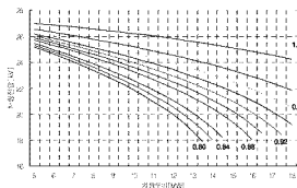
그림 9. 부하, 역률에 따른 차량의 집전곡선
