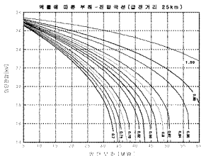
그림 3. 급전선로 P-V 곡선(급전거리 25km)
