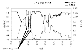
그림 8. 변전소 급전측 전압 및 전류
