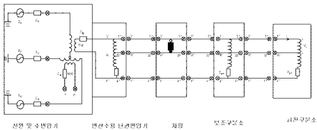
그림 1. 교류 급전시스템의 구성
