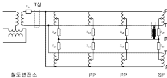
그림 2. 전압안정도 예측계산을 위한 급전계통
