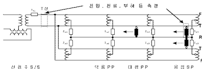
그림 5. 급전계통 전력전송능력 추정을 위한 차량위치
