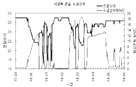
그림 6. 선로말단 차량측 전압 및 소모부하
