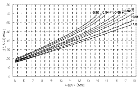
그림 12. 부하, 역률에 따른 변전소 공급부하
